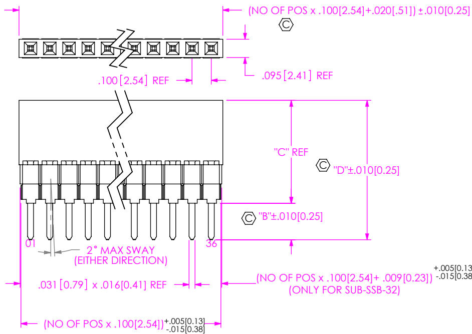
FIG 1 ESW-1XX-XX-X-S SHOWN
