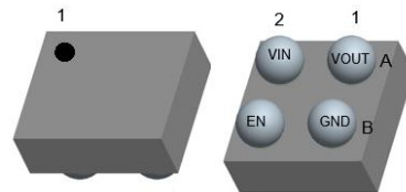
0.77 mm x 0.77 mm x 0.46 mm WLCSP
