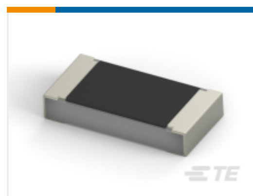
TE 产品编号3-2176230-9 SMD 功率电阻器：3 瓦特，5% Tol
