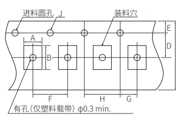
F=4mm (105、21、316、32 封装)
