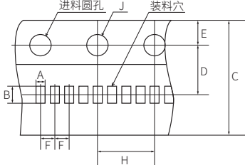
F=1mm (02、03、05 封装)
