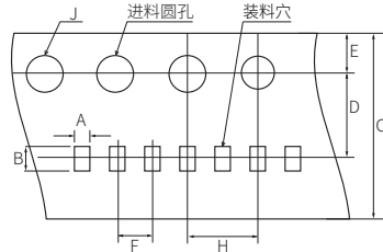
F=1mm (02 封装)
