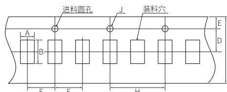
F=2mm (02、03、05 封装)
