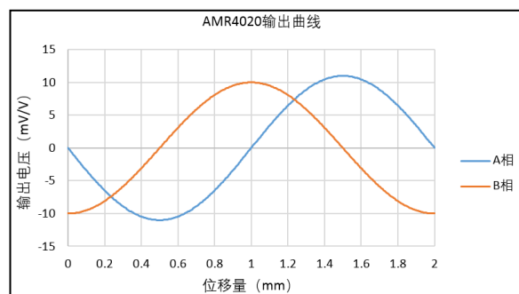
图 4 AMR4020 沿磁栅长度方向移动时的输出电压
