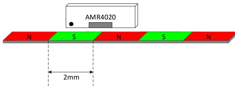
图 3 AMR4020 与磁栅相对位置
