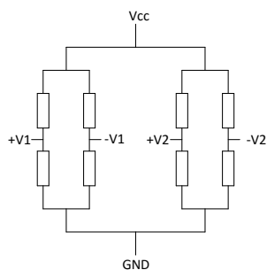
图 2 电气原理图
