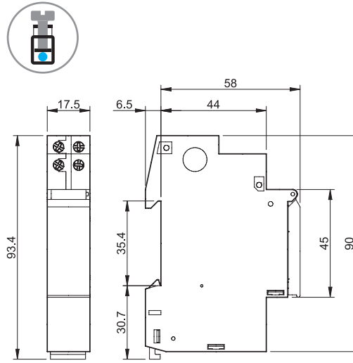
12.11 螺絲終端
