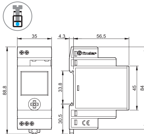
12.51/12.81 螺絲終端
