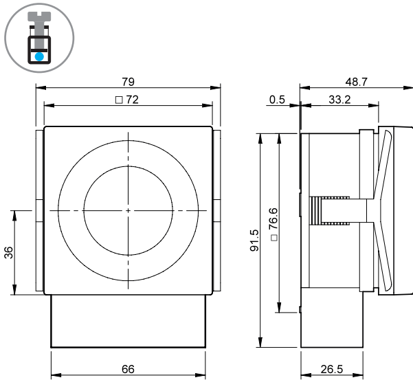
12.31 螺絲終端
