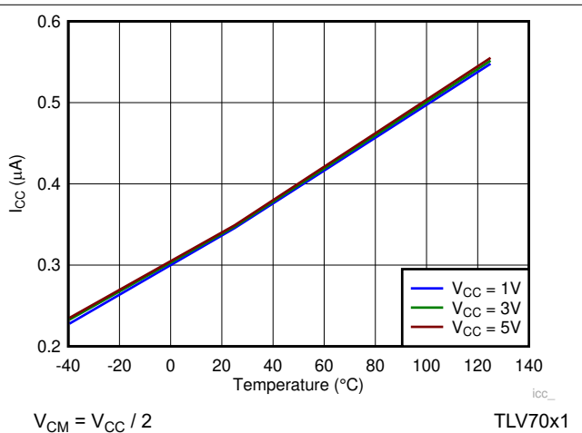
图 6-26. I_{CC} vs Temperature
