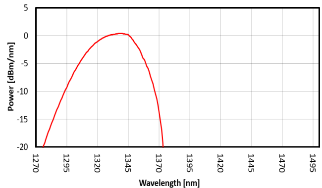
FIG. 4: SLED 3 SPECTRUM
