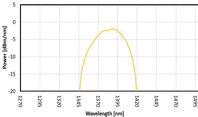
FIG. 3: SLED 2 SPECTRUM
