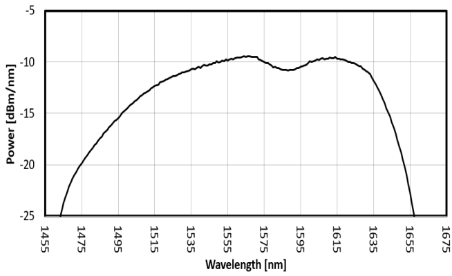
FIG. 1: OSE2 SPECTRUM
