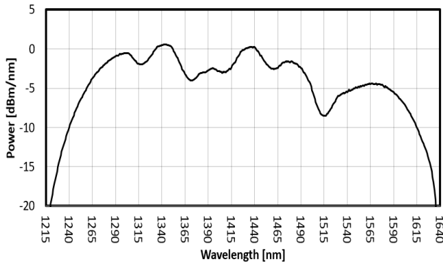
FIG. 1: OSE2 SPECTRUM
