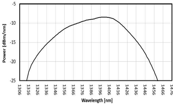
FIG. 1: ISB1 SPECTRUM
