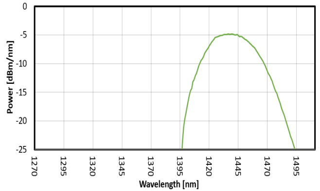
FIG. 2: SLED 1 SPECTRUM
