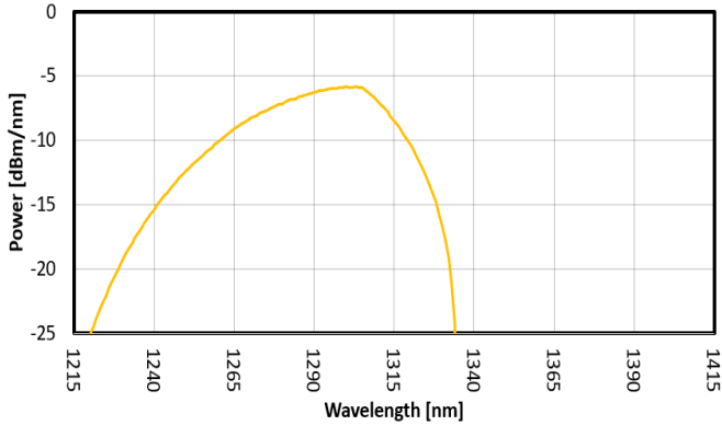
FIG. 3: SLED 2 SPECTRUM
