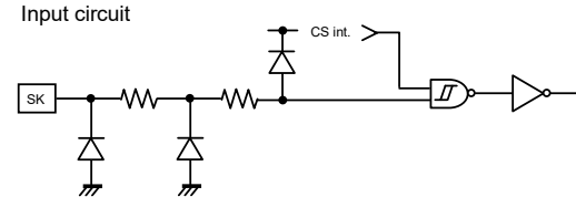
Figure 47. Input circuit (SK)
