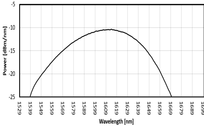
FIG. 1: ISB1 SPECTRUM
