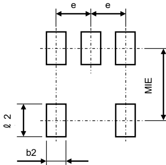
SSOP5
