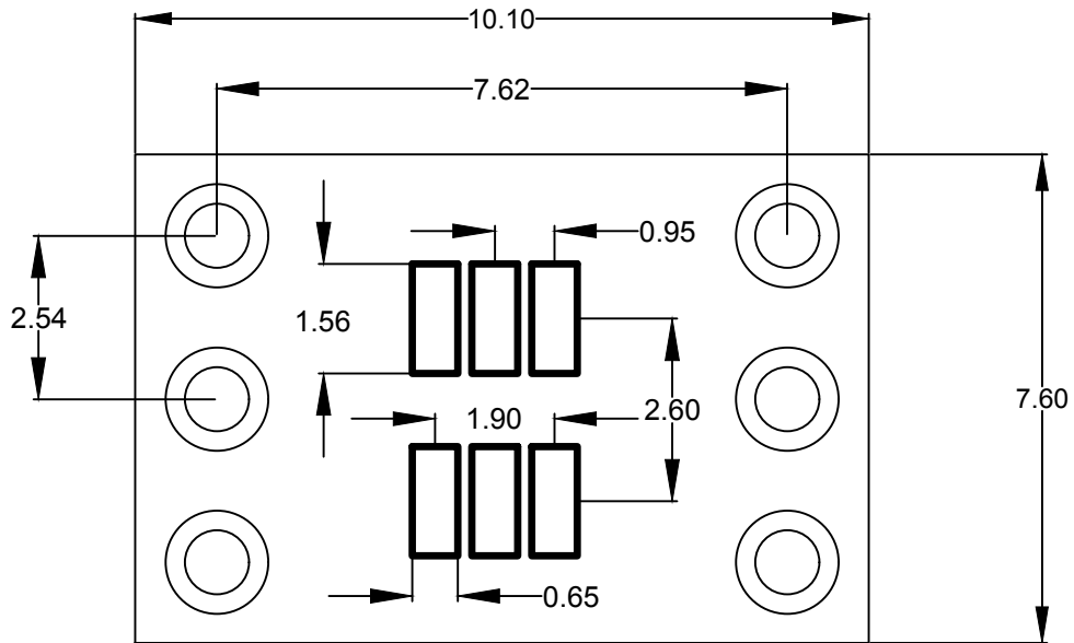
Front: SOT23-6
